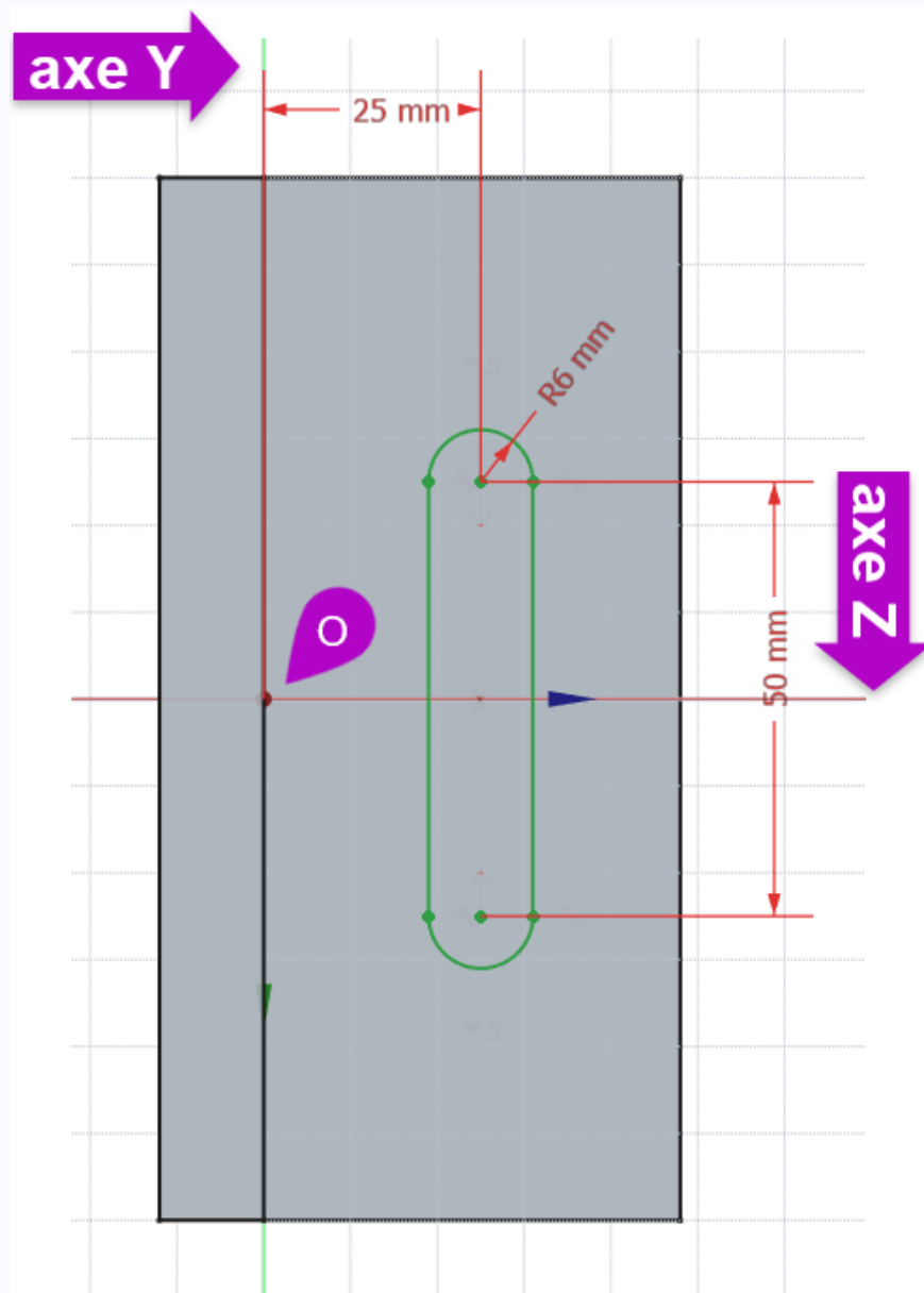
Esquisse n°2 pour le trou oblong
