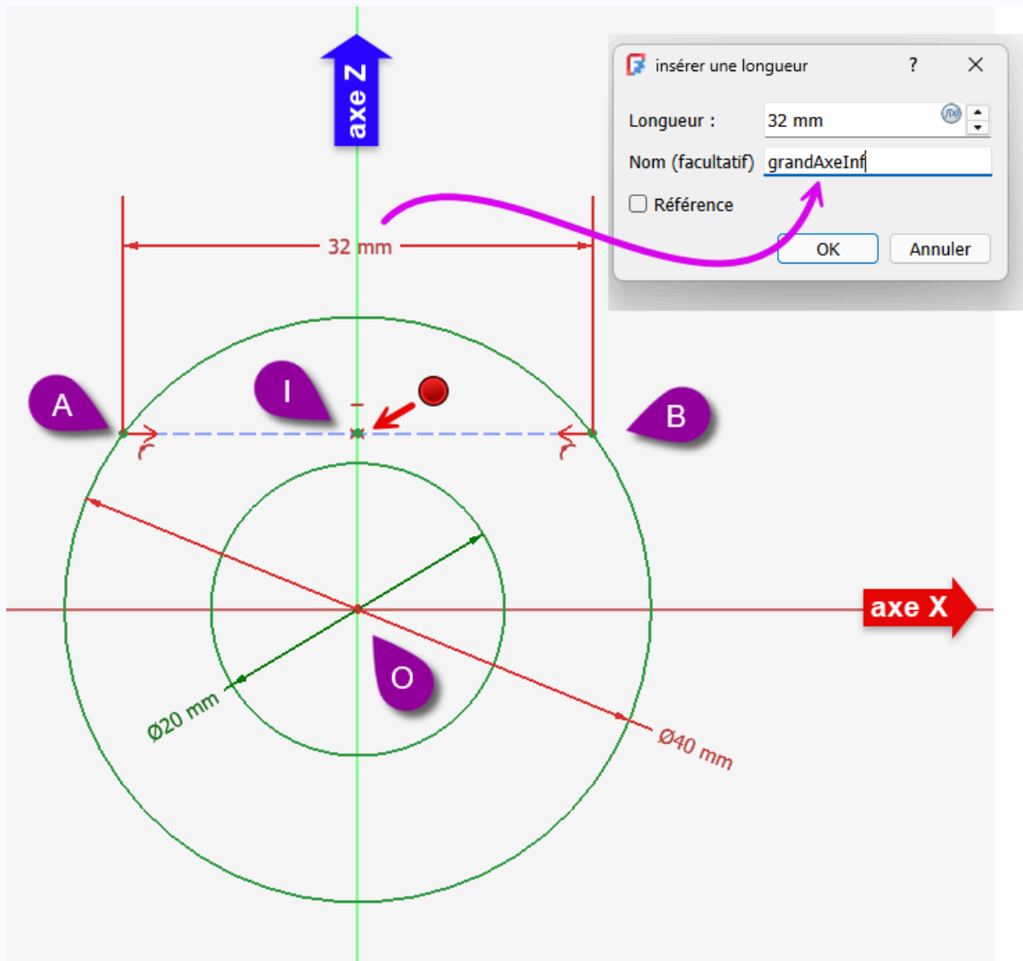
Esquisse du cylindre inférieur
