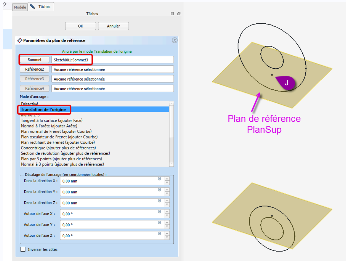
Plan de référence pour le haut de la nervure
